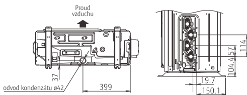
Pohled zdola
