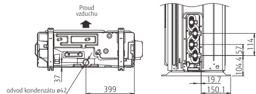
Pohled zdola
