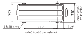
Pohled shora
